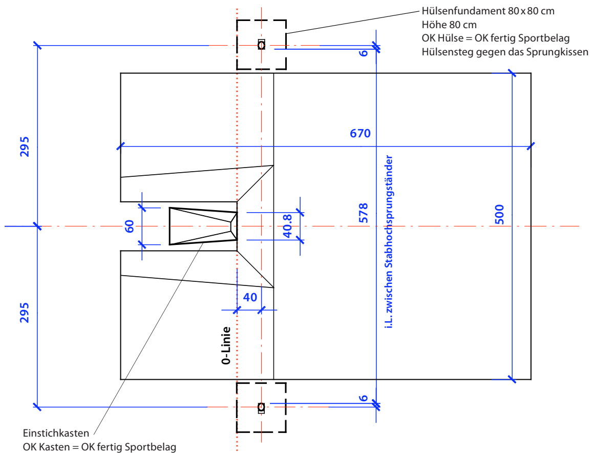
Draufsicht
